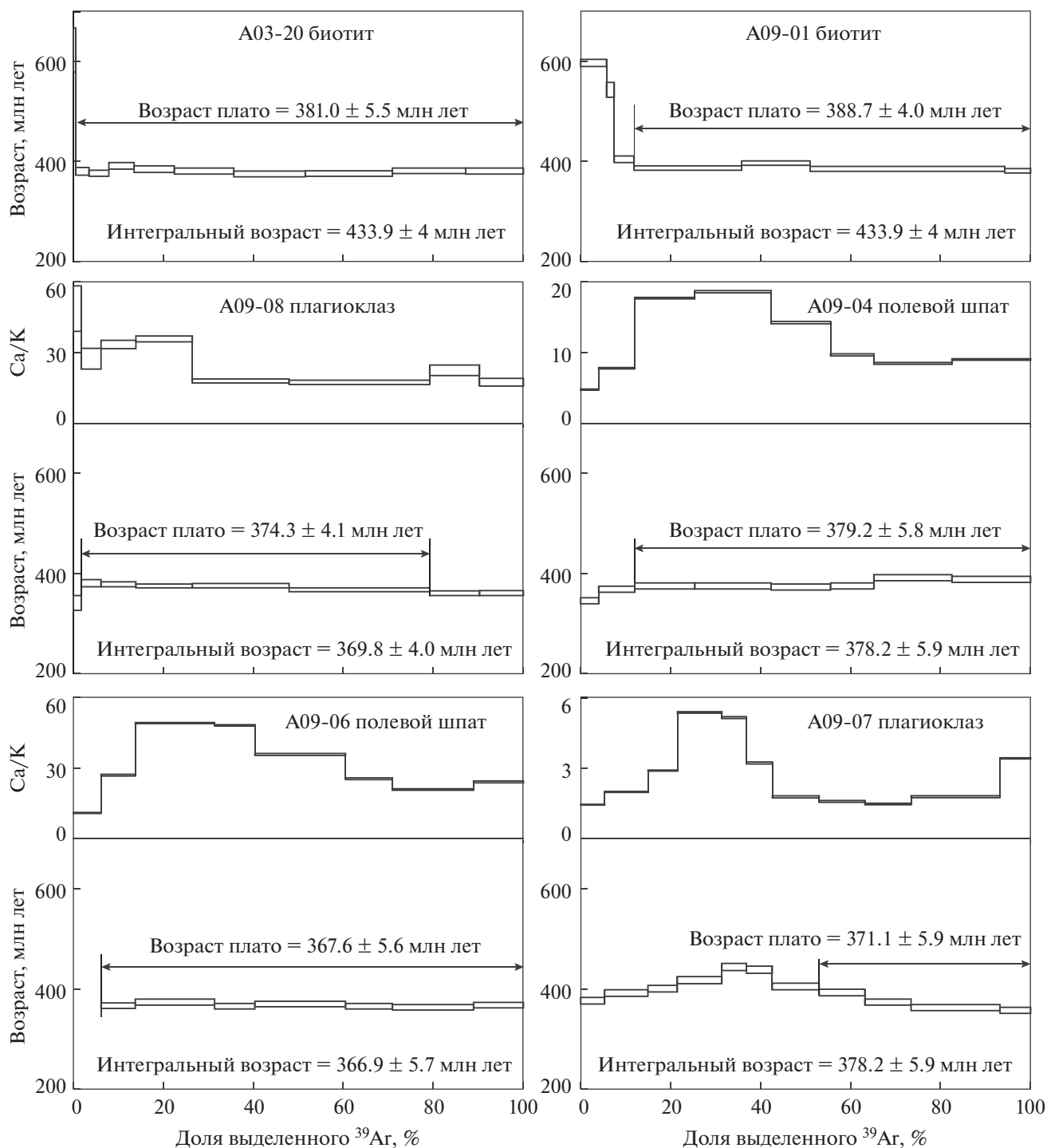
Рис. 4. Результаты ^{40}\text{Ar}/^{39}\text{Ar} исследований методом ступенчатого прогрева монофракций биотита и плагиоклаза из долеритов печенгского и баренцевоморского роев даек. Координаты проб: A03-20 – 69^{\circ}30'08'' с.ш., 31^{\circ}15'30'' в.д., A09-01 – 69^{\circ}07'24'' с.ш., 36^{\circ}02'55'' в.д., A09-08 – 69^{\circ}11'38'' с.ш., 35^{\circ}07'43'' в.д., A09-04 – 69^{\circ}06'22'' с.ш., 36^{\circ}03'47'' в.д., A09-06 – 69^{\circ}07'08'' с.ш., 36^{\circ}06'27'' в.д., A09-07 – 69^{\circ}07'09'' с.ш., 36^{\circ}06'28'' в.д. (Система координат WGS84).
