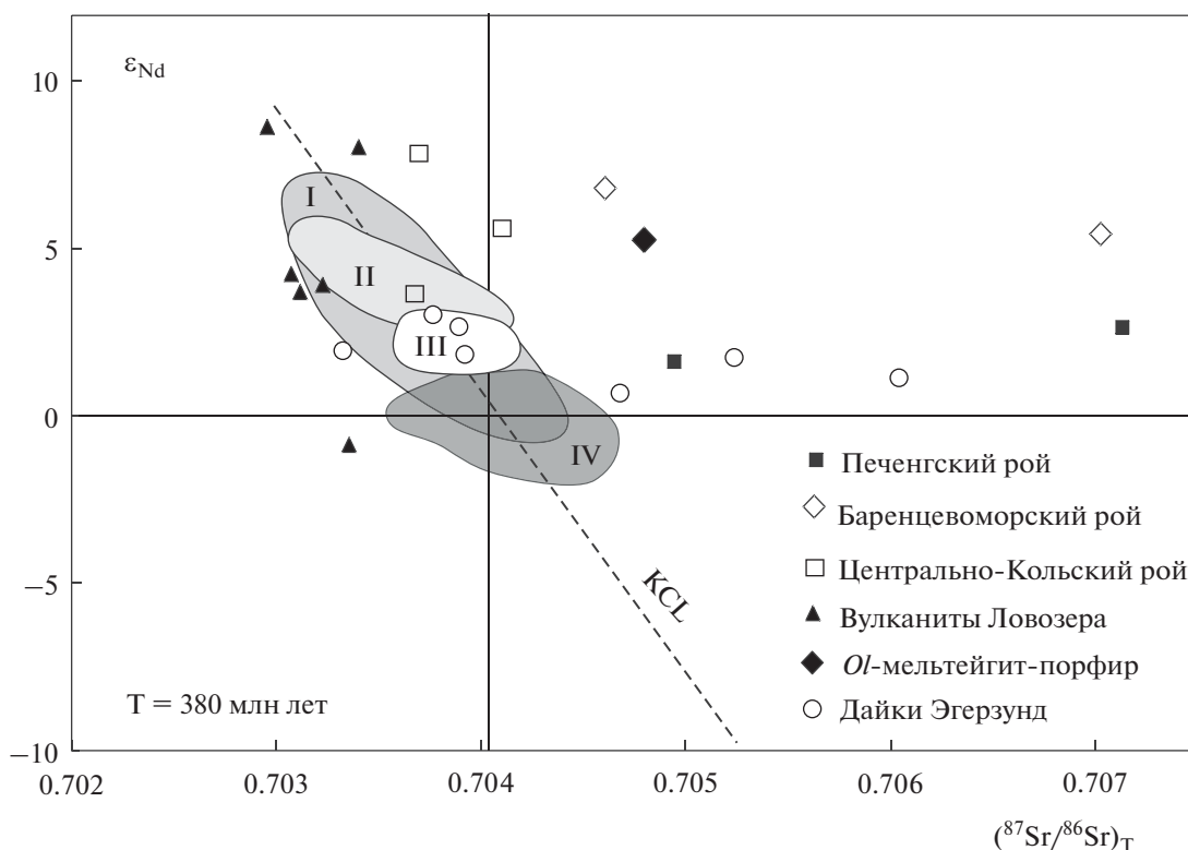
Рис. 7. Диаграмма распределения значений (^{87}\text{Sr}/^{86}\text{Sr})_T и \epsilon_{\text{Nd}}(T) в палеозойских долеритах и вулканитах Ловозерского массива. Для сравнения полями показаны области изотопных составов пород щелочно-ультраосновных интрузий Кольской провинции (I), Хибинского (II) и Ловозерского (III) массивов, палеозойских щелочных пород дайковой серии (IV), по данным (Amelin, Zaitsev, 2002; Downes et al., 2005; Арзамасцев и др., 1999; 2009; Kramm et al., 1993; Kramm, Kogarko, 1994; Rukhlov, Bell, 2010; Wu et al., 2010), а также даек района Эгерзунд, по (Bingen, Demaiffe, 1999). KCL — “Кольская карбонатитовая линия смешения” по (Kramm et al., 1993).
