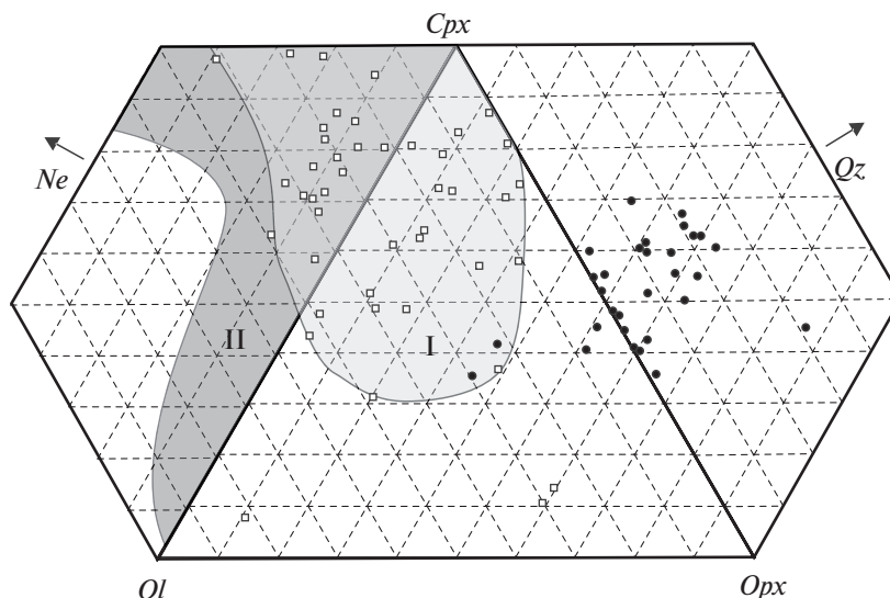
Рис. 8. Диаграмма нормативных составов палеозойских долеритов и вулканитов Ловозерского массива в координатах нефелин (Ne) — клинопироксен (Cpx) — кварц (Qz) — ортопироксен (Opx) — оливин (Ol). Залитые кружки — породы палеозойской толеитовой серии, незалитые квадраты — субщелочные и щелочные вулканиты ловозерской серии, полями показаны области нормативных составов пород щелочно-ультраосновных интрузий Кольской провинции (I), Хибинского и Ловозерского массивов (II).
